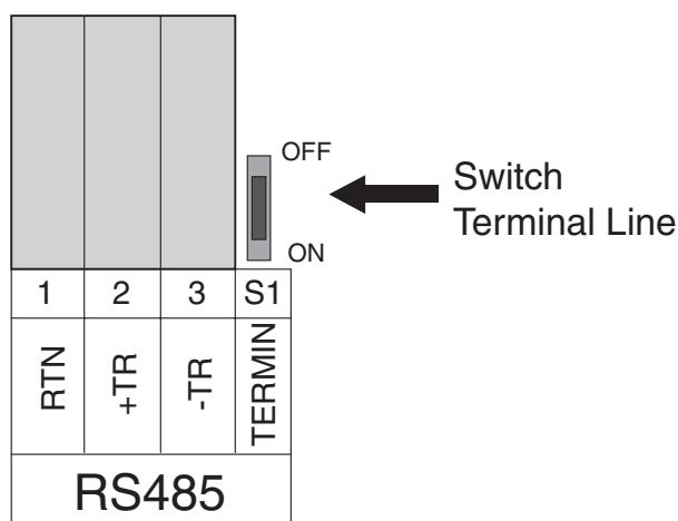
Abb. 17: Klemmenblöcke des seriellen Anschlusses RS-485
