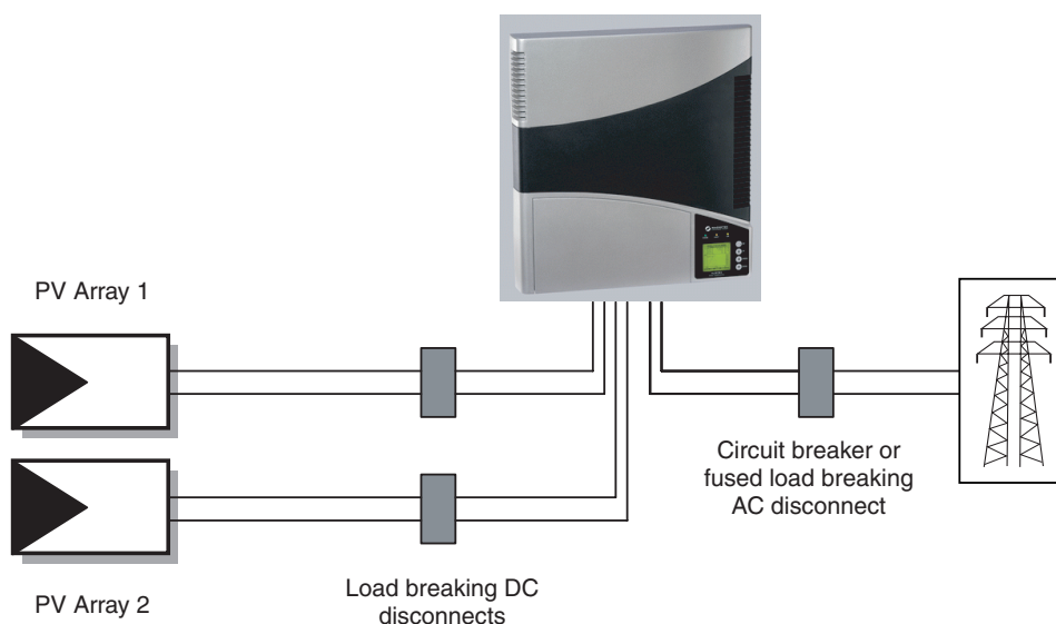
Abb. 3 Vereinfachtes Schema eines Photovoltaik-Systems
