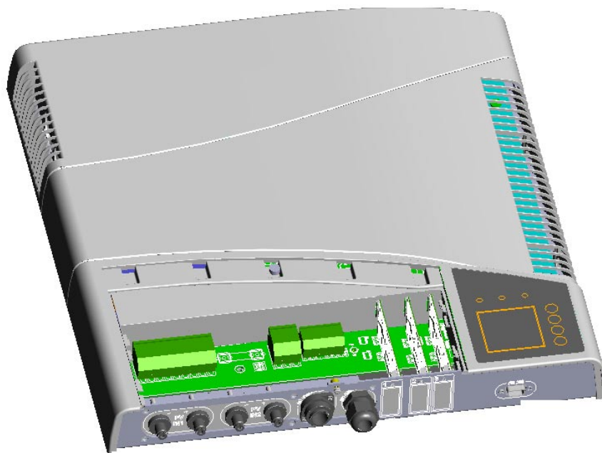
Abb. 9 Anschlüsse an der Unterseite des Wechselrichters
