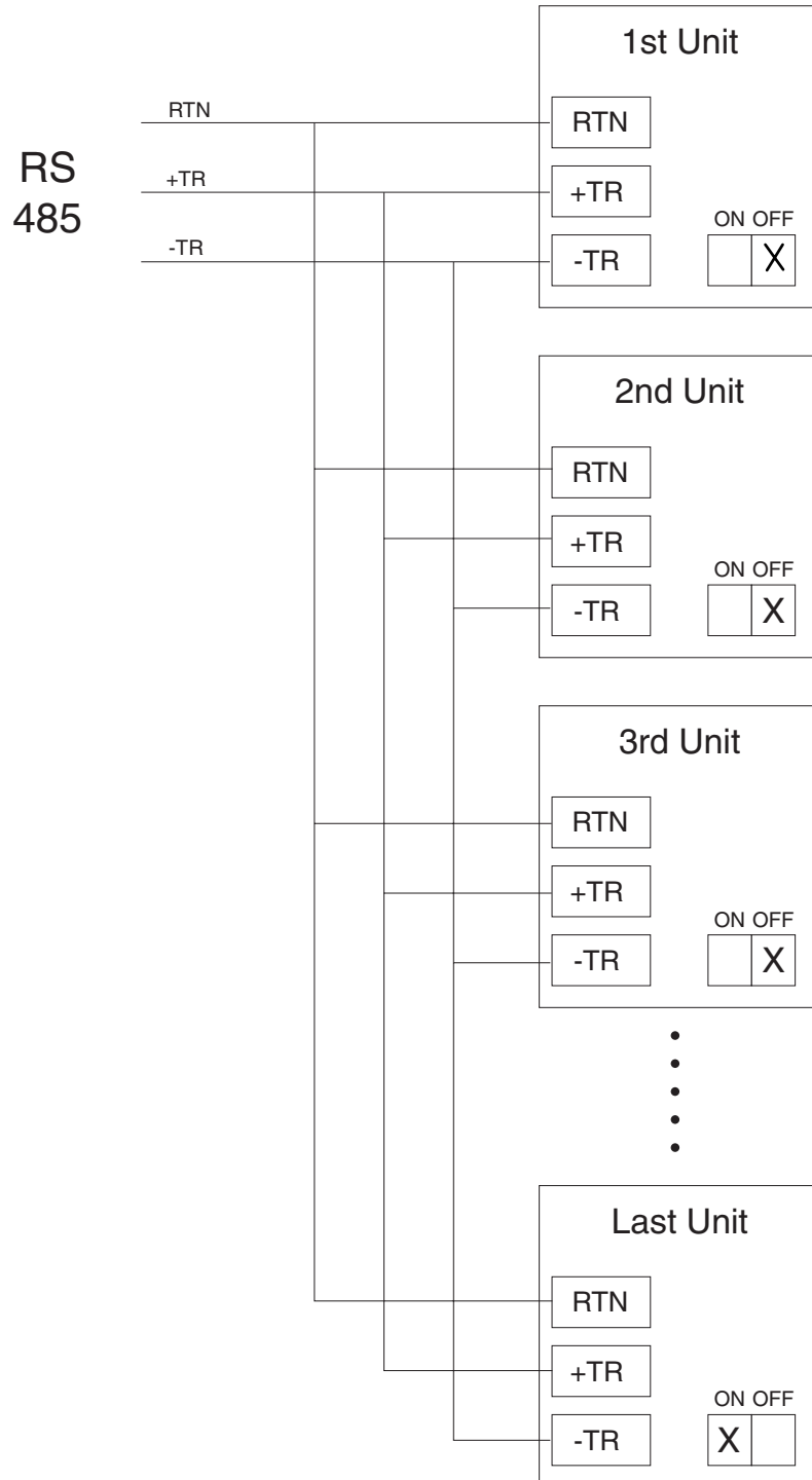
Abb. 18 Mehrfachschaltung vom Typ "daisy-chain"
