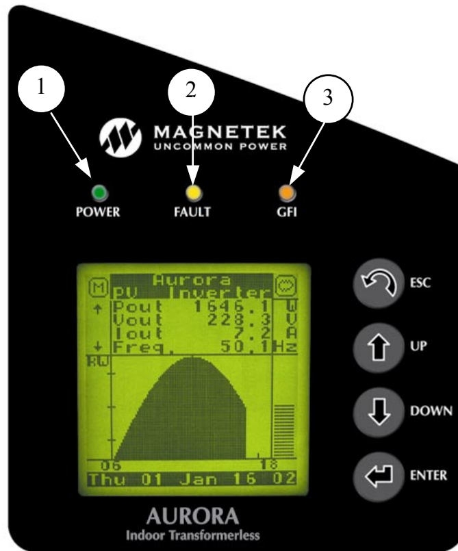
Abb. 15 LED - Anzeige
