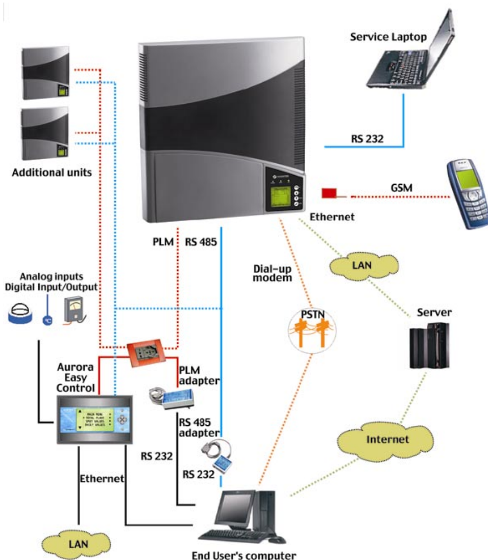
Abb. 19 Datenübertragung an das Aurora Easy Control-System
