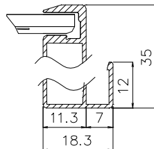
Abschnitt A-A'
