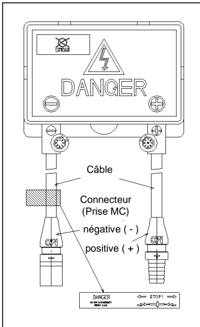
Figure 3: Configuration de la boîte de connexion
