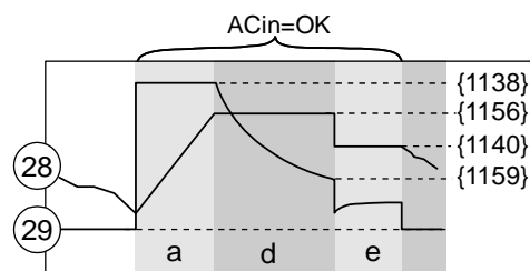
Fig. 3b: Vereinfachter Batterieladezyklus ohne Eingangsstrombegrenzung
